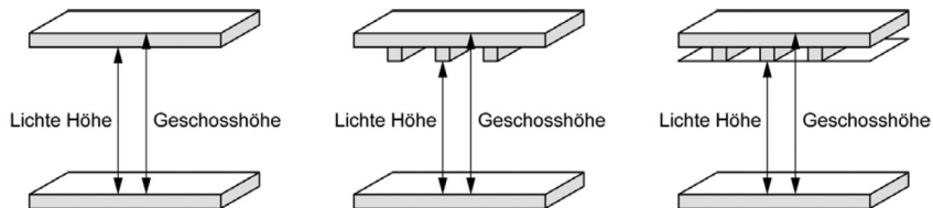
Figur 5.4 Lichte Höhe
