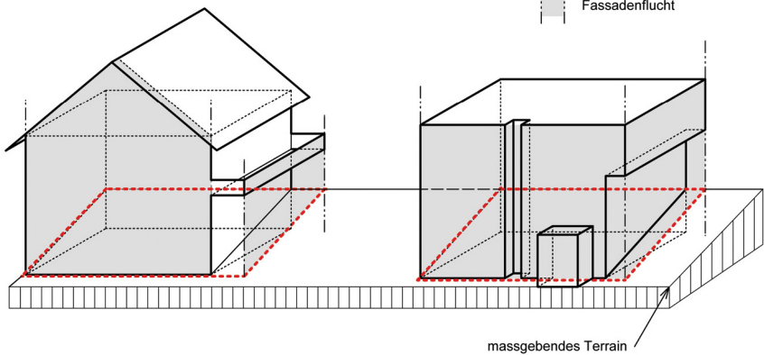
Figur 3.1 – 3.3 Fassadenflucht und Fassadenlinie
