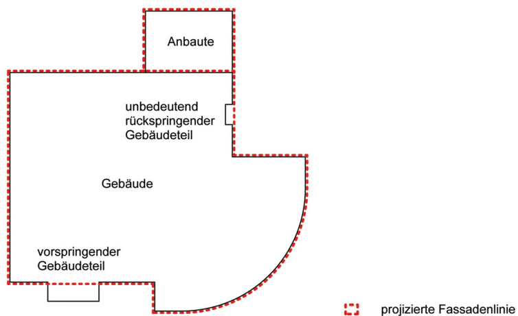
Figur 3.3 Projizierte Fassadenlinie
