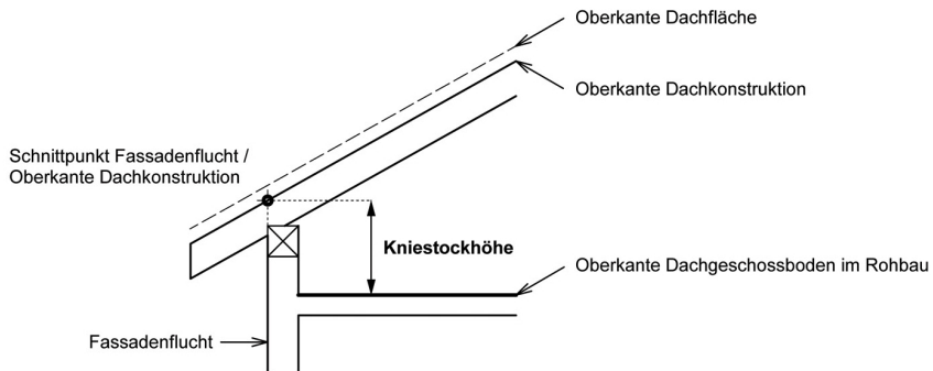
Figur 5.3 Kniestockhöhe
