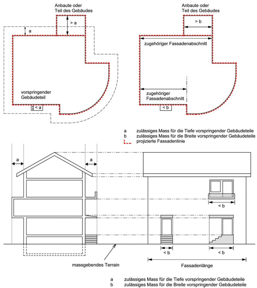
Figur 3.4 Vorspringende Gebäudeteile (Schnitt und Seitenansicht)
