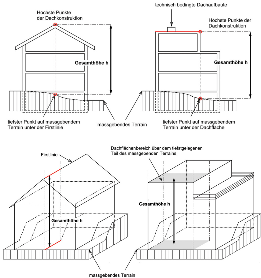
Figur 5.1 Gesamthöhe
