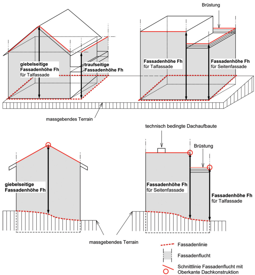
Figur 5.2 Fassadenhöhe
