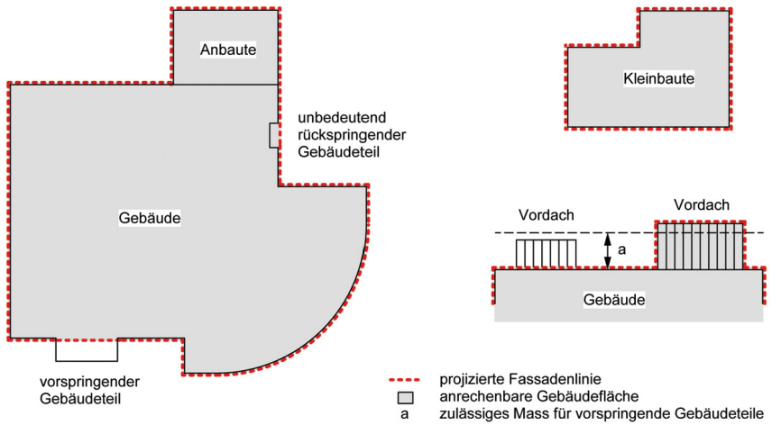
Figur 8.4 Anrechenbare Gebäudefläche
