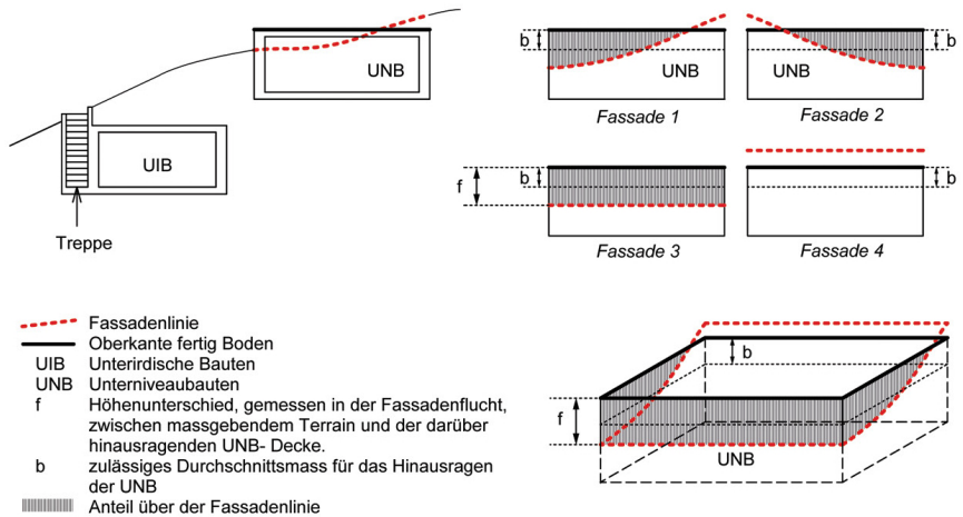
Figur 2.4 und 2.5 Unterirdische Bauten, Unterniveaubauten
