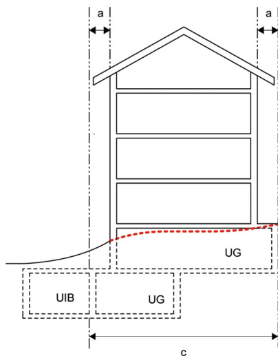
Figur 6.2 Untergeschosse
